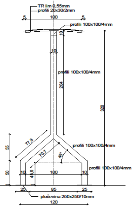
POPREČNI PRESEK NOSAČ TENDE
