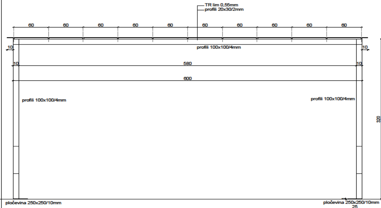
PODUŽNI PRESEK NOSAČ TENDE
