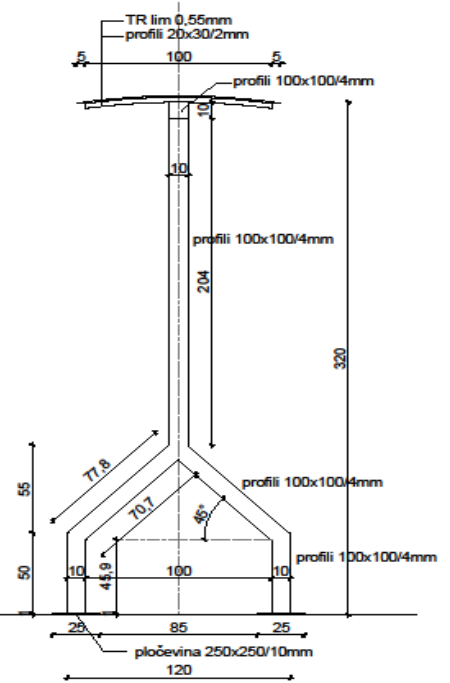
POPREČNI PRESEK NOSAČ TENDE
